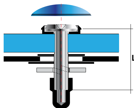
Abb. Aufbau und Abmessungen der Balkonschraube
